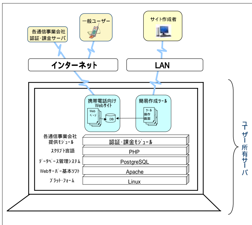
ユーザー環境に配置した場合のシステム構成図
