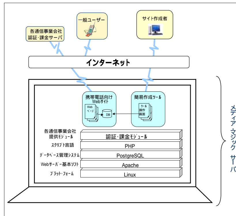
メディア・マジック内に配置した場合のシステム構成図
